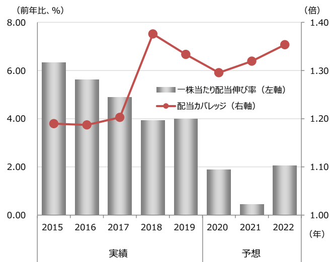
図2：中流MLPの配当伸び率と配当カバレッジ
