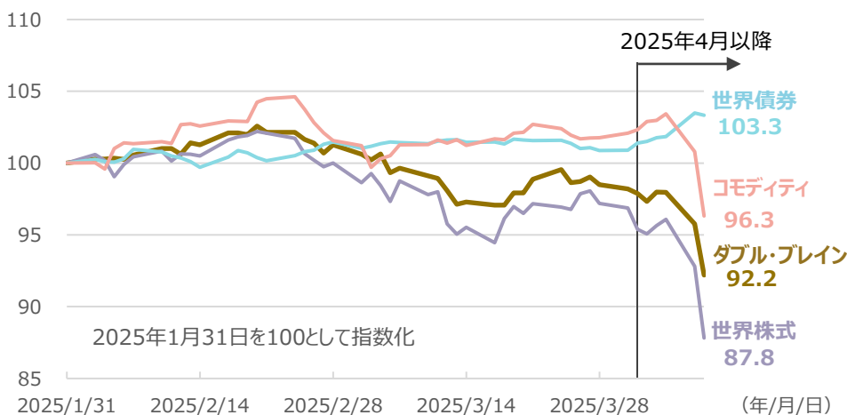
ダブル・ブレインと各指数（円ヘッジベース）のパフォーマンス推移
